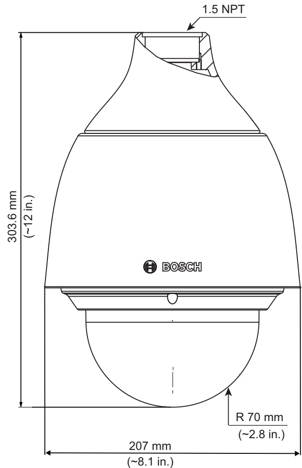
Fig. 5: Pendant model
